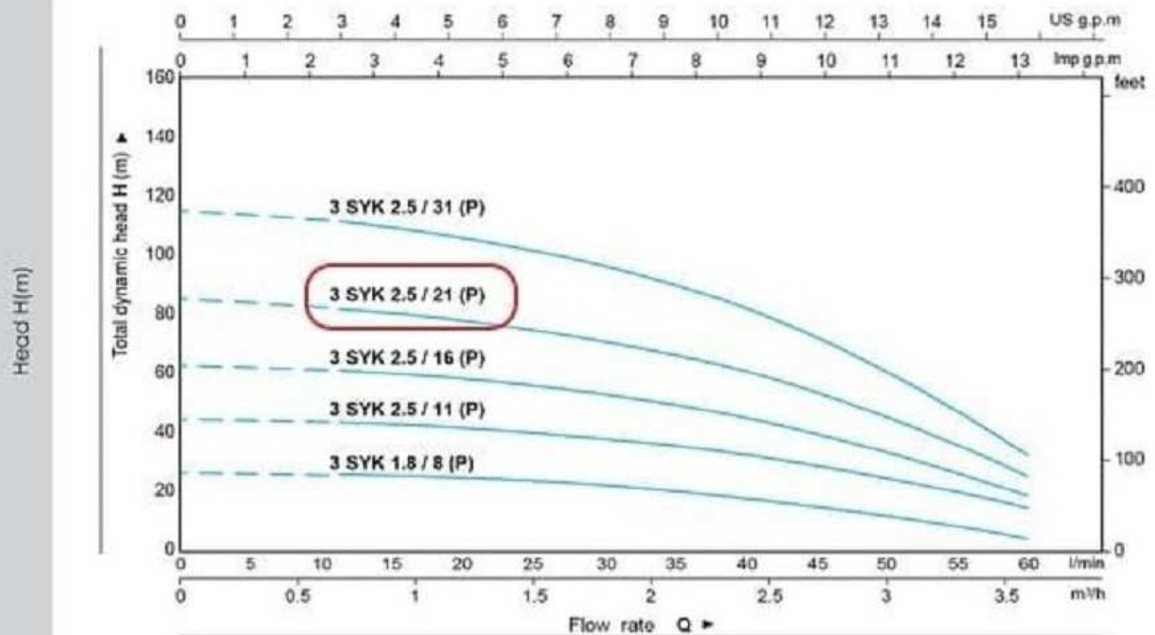
Capacity Q(M³/h)
